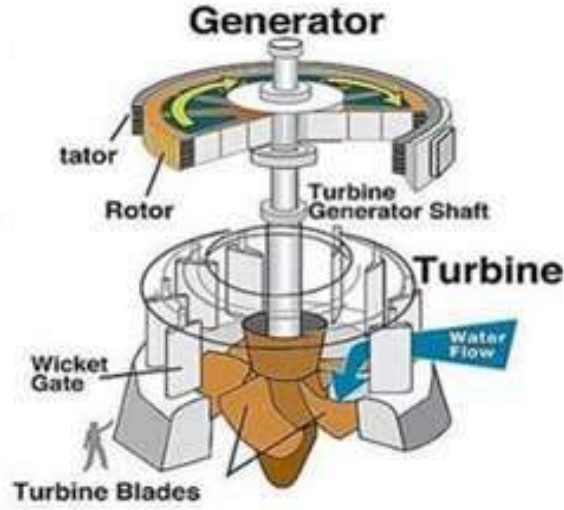
Örnek Bir Türbin – Generatör kesiti (*)
