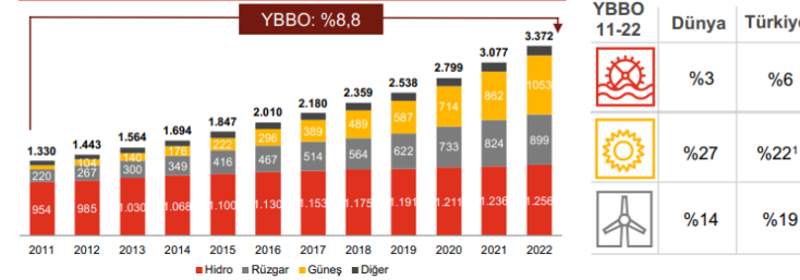
Küresel Yenilenebilir Enerjinin Kurulu Gücü (2011-2022, GW)
