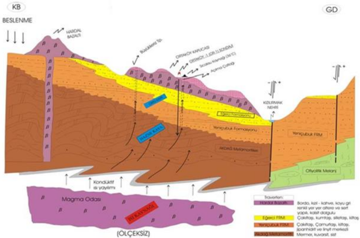
Şekil: Ortaköy jeotermal sahasının modeli
